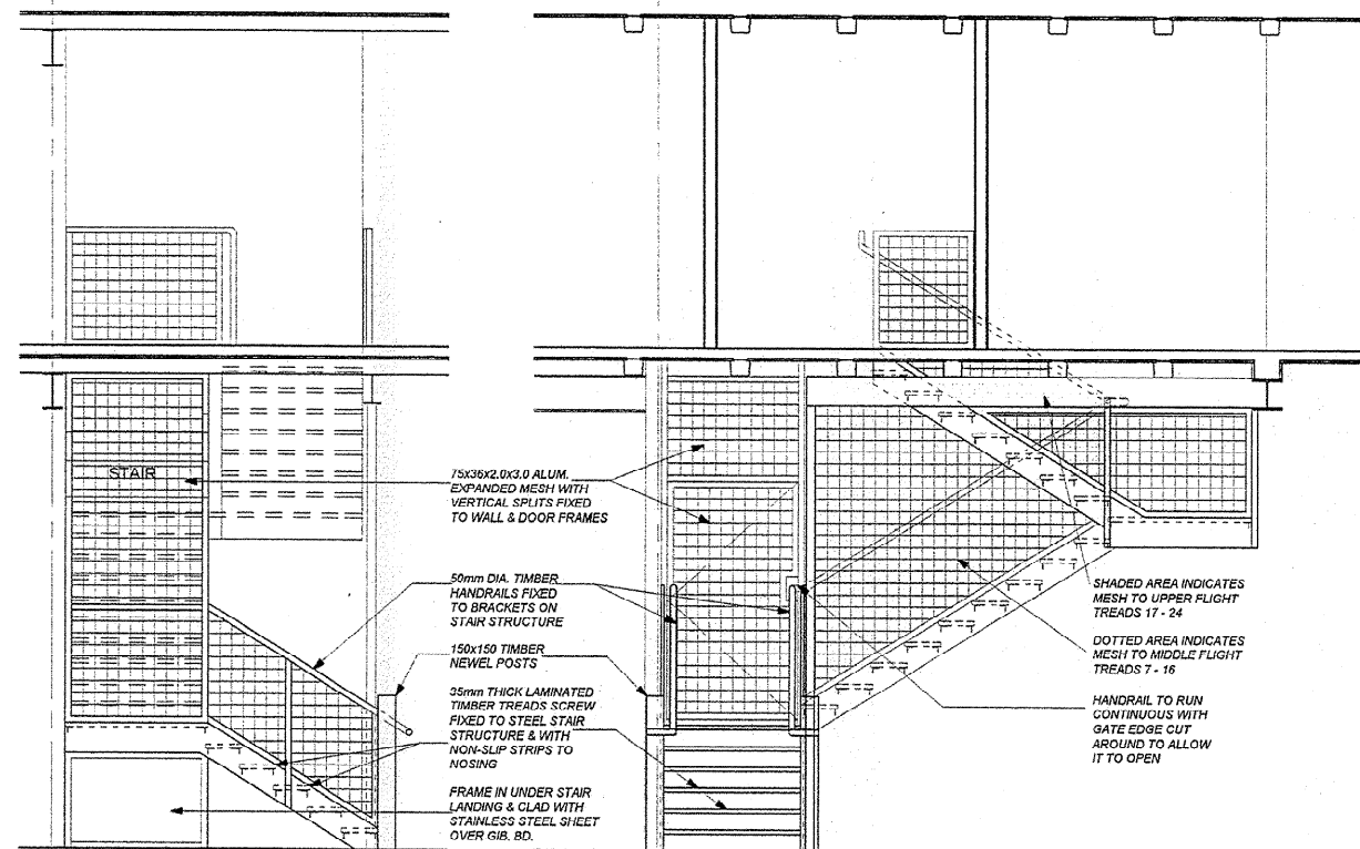
ELEVATION A
