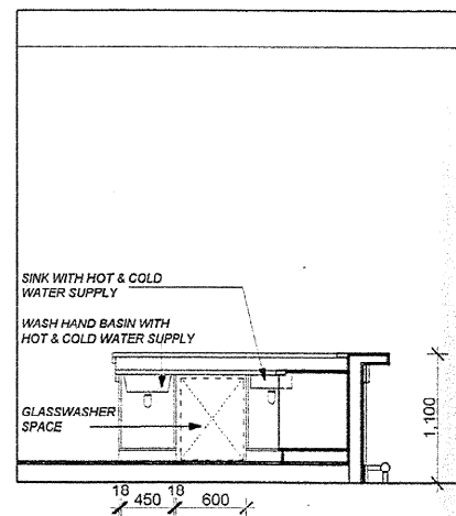
ELEVATION 1
