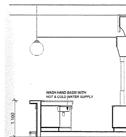
ELEVATION 3
