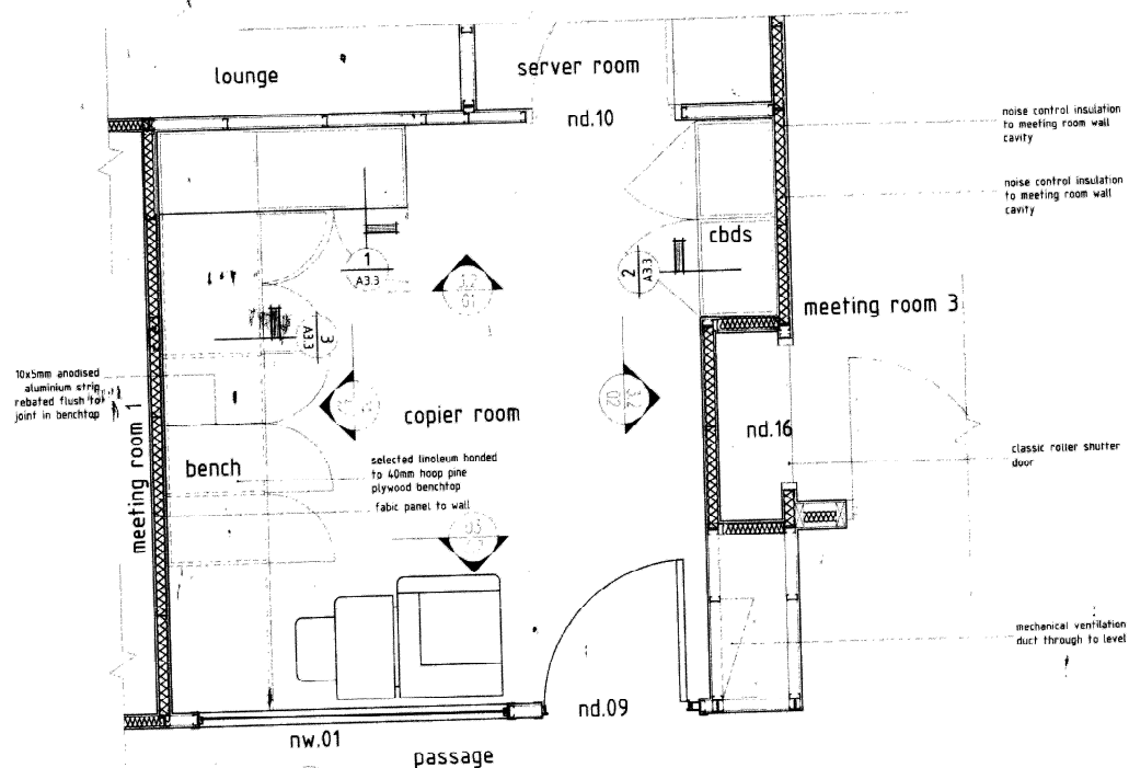
Copier Room Plan 01 125 A3.3
